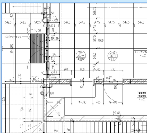
<平面詳細図>
