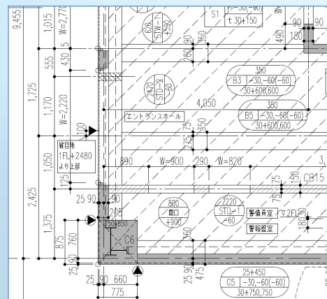
<躯体図>
