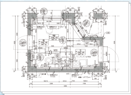
平面詳細図
