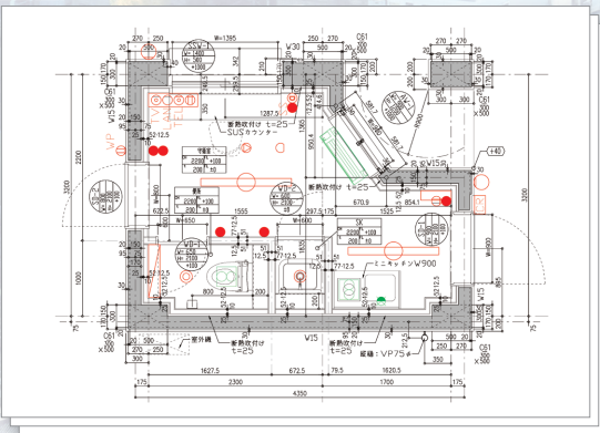
総合図(電気・空調・衛生)
