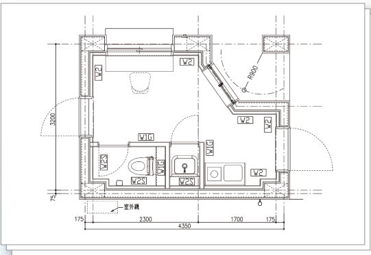
意匠図
