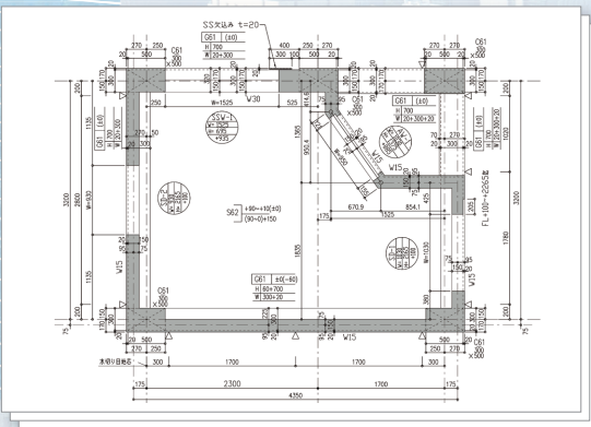
躯体図
